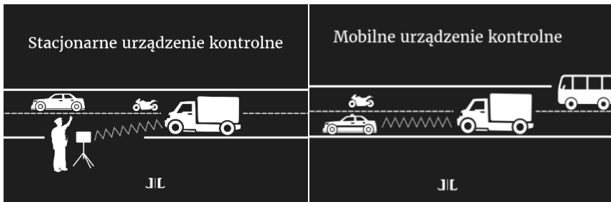
Rys.2. Schemat działania zdalnej kontroli przy użyciu DSRC [1]
