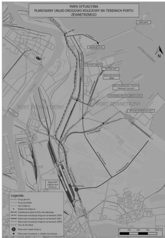
Rys. 2. Planowana układ sieci drogowo-kolejowej w Porcie Gdańsk
