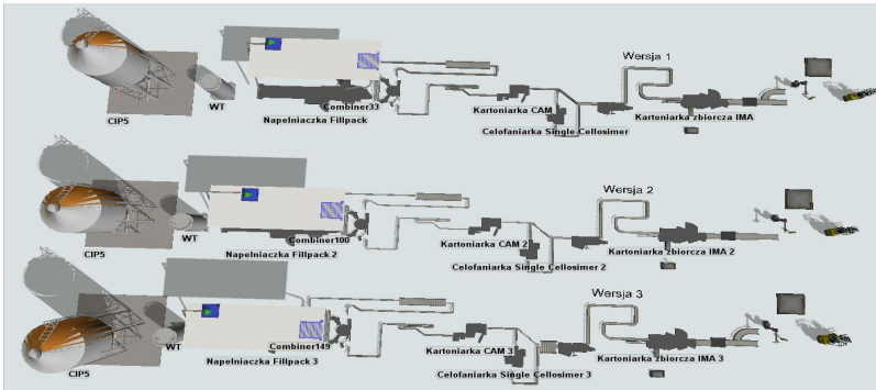
Rys. 14. Modele linii produkcyjnej.
