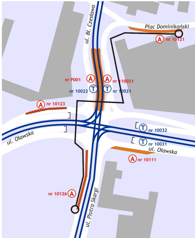
Rys. 4. Droga dojścia pasażera pomiędzy dwoma skrajnymi punktami na węzle przesiadkowym według koncepcji pierwszej.
