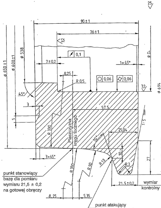
Rys. 1. Profil PST według normy PN-K-92016.
