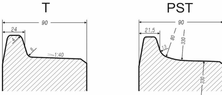
Rys. 6. Zarysy obręczy tramwajowych T i PST. Źródło: opracowanie własne.
