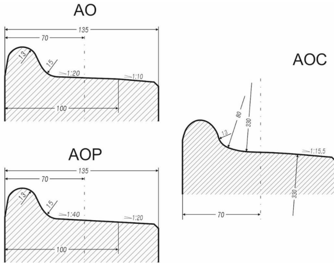
Rys. 5. Zarysy obręczy kolejowych AO, AOP, AOC. Źródło: opracowanie własne.
