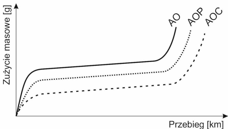
Rys. 4. Poglądowy przebieg zużycia ściernego obręczy w funkcji przebiegu.
